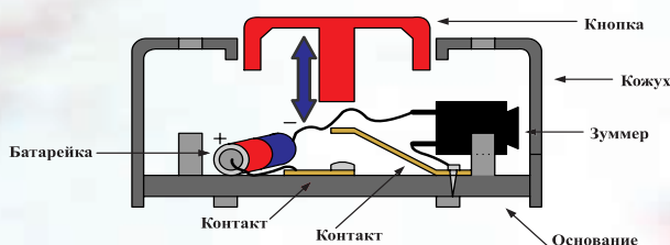
Рис. 2 Кнопка звонка со звуковой реакцией на нажатие
