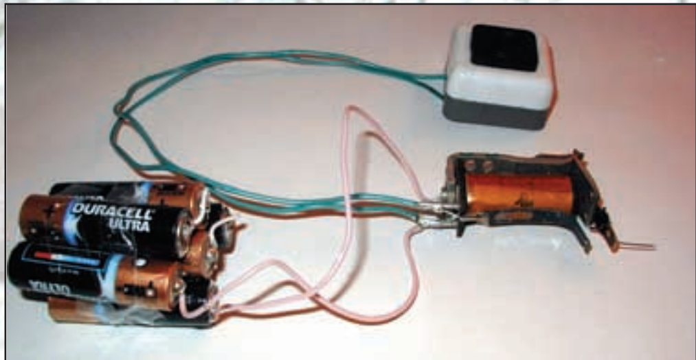
ЕСЛИ СОБРАТЬ ЭЛЕКТРИЧЕСКУЮ ЧАСТЬ, ТО ЭТО БУДЕТ ТАК. ЗДЕСЬ В СЕВШИХ БАТАРЕЕК ДЛЯ НАДЕЖНОСТИ. ХОТЯ ХВАТАЕТ ТРЕХ.
