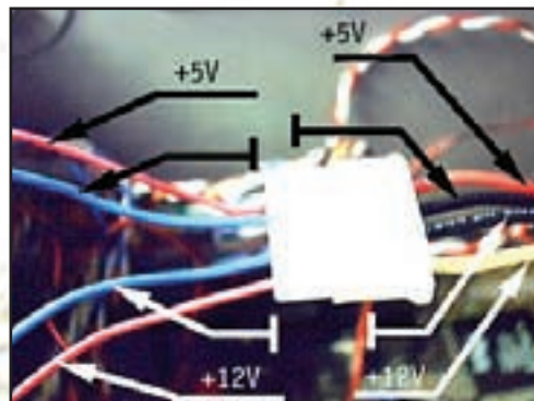
КРАСНЫЙ ПРОВОД - +5V ЧЕРНЫЙ ПРОВОД - КОРПУС ЖЕЛТЫЙ ПРОВОД - +12V
