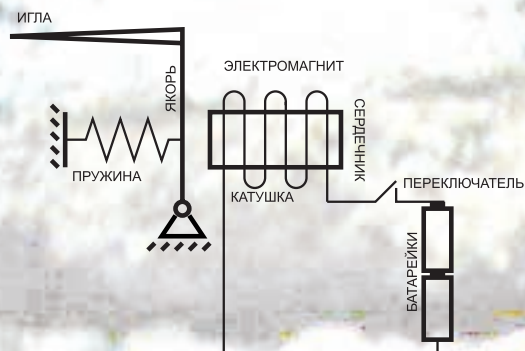
Исходное состояние схемы пускателя
