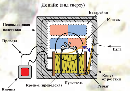
ЭЛЕКТРИКУ НУЖНО УПАКОВАТЬ В КОРПУС ПО ТАКОЙ СХЕМЕ
