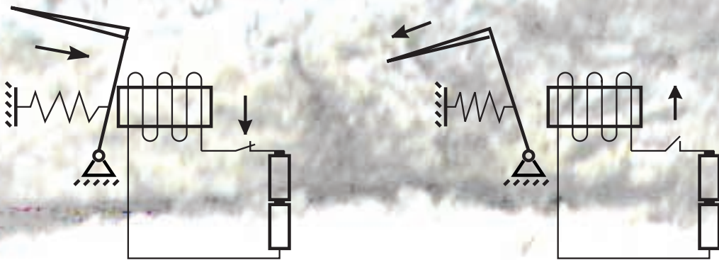
Размыкаем переключатель, электромагнит отпускает якорь, пружина с силой выбрасывает иглу.
