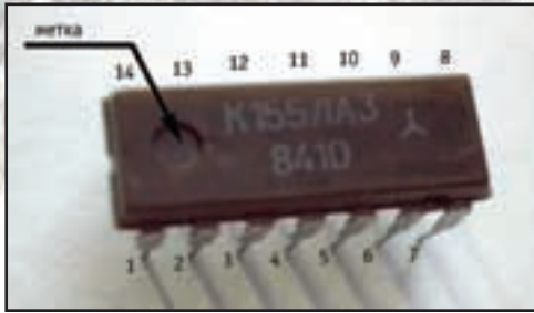
ОПРЕДЕЛЕНИЕ ВЫВОДОВ МИКРОСХЕМЫ
